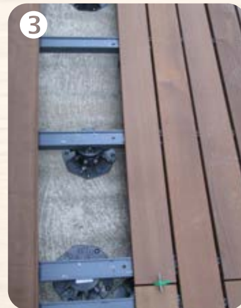
TERRASSEN AUFBAU Der Unterbau ist für eine dauerhafte Terrasse ausschlaggebend.
